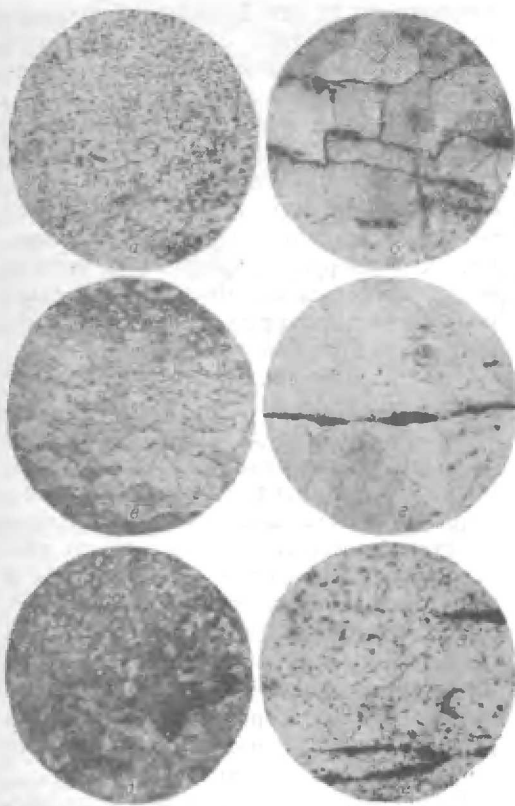
Рис. 2. Микроструктура металла меча:
