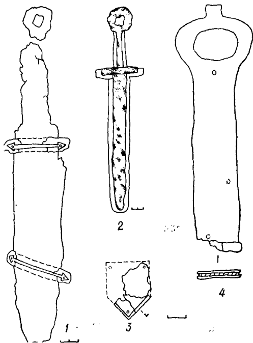
Рис. 8. Оформление ножен и рукоятей: 1 — Усть-Каменка, 4/1; 2 — Старые Куканешты; 3 — Новофилипповка, северная группа 1; 4 — Новофилипповка 2 (раскопки М. Я. Рудинского).
